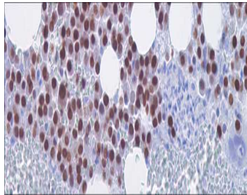
Tonsil
